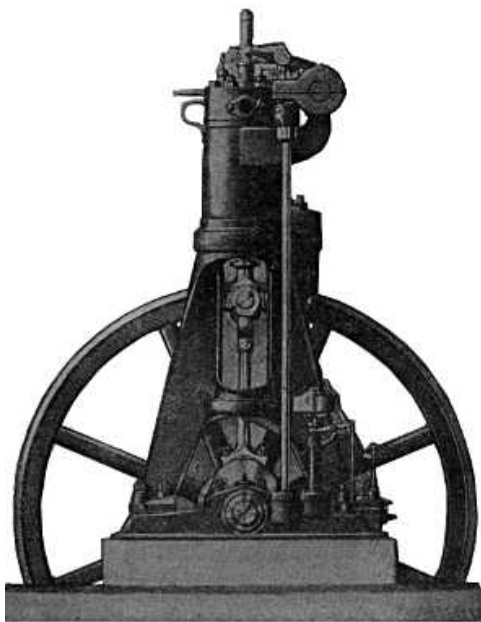
Современный судовой двигатель Дизеля в 60 лш. сил завода «Бр. Зульцер»
