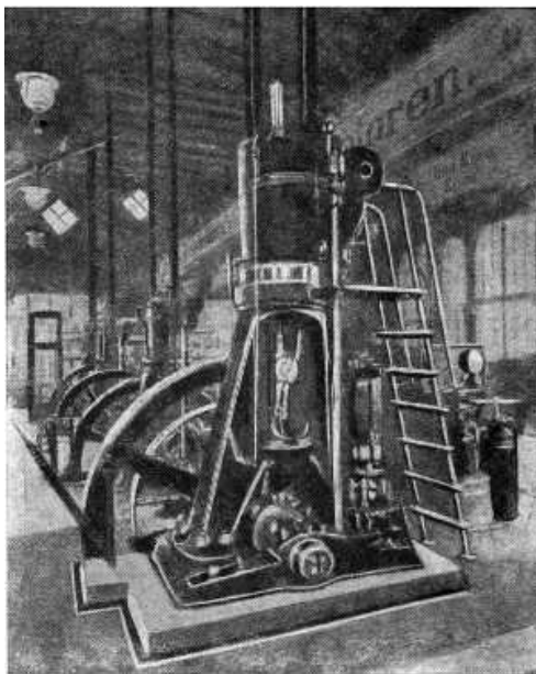
Двигатели на Мюнхенской выставке 1898 года
