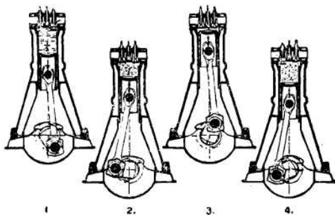
Схема работы, двигателя Дизеля: 1 — всасывание; 2 — сжатие; 3 — рабочий ход; 4 — выхлоп
