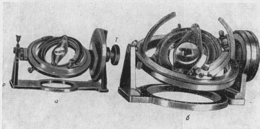
Федоровский столик: а) ранняя конструкция, б) современная.
