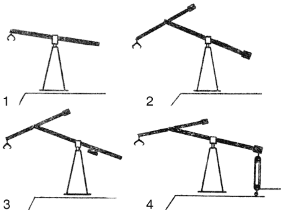
Рис. 2. Возможные схемы оборонительной машины Архимеда
