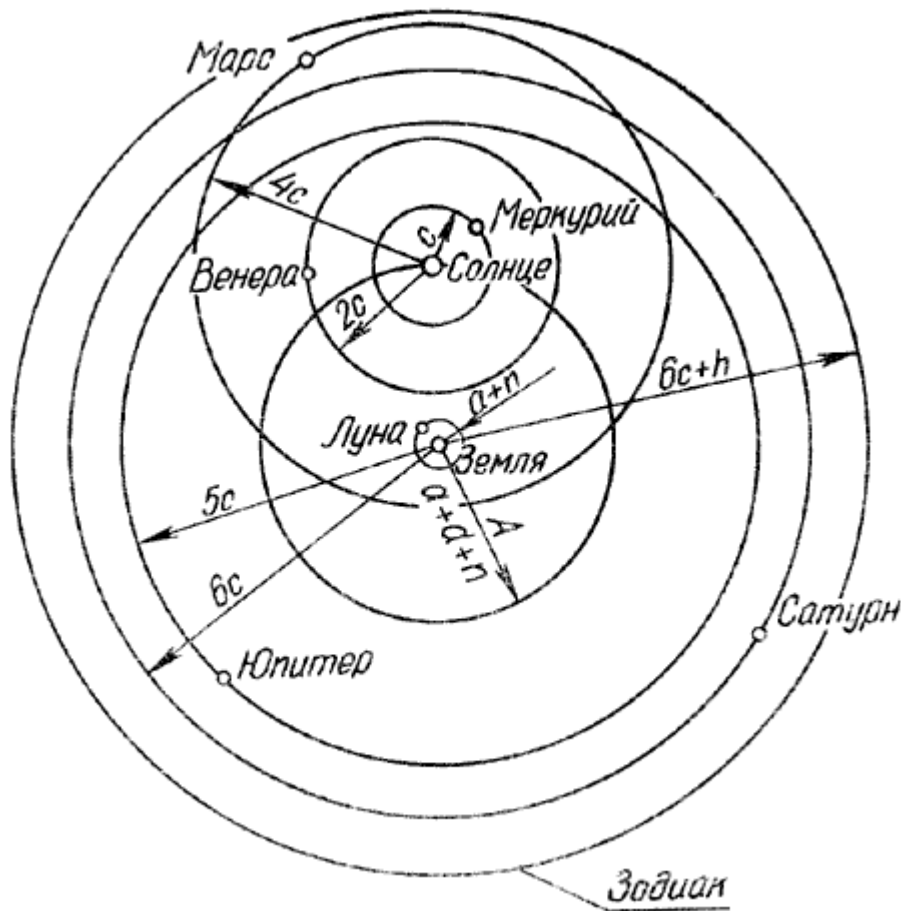
Рис. 6. Система мира Архимеда (указаны межпланетные расстояния в мириадах стадий). a = 554 , d = 5081 , A = 5640 , c = 2027 , h = 2007 , n = 4
