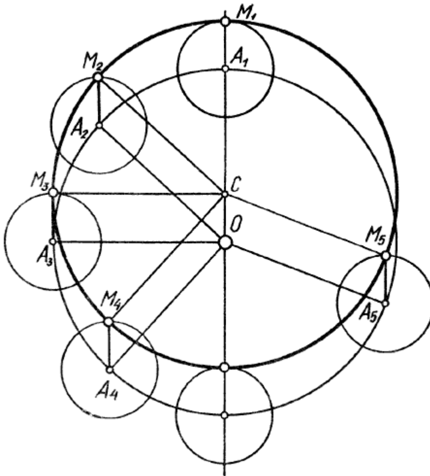
Рис. 3. Изображение перемещений «верхней» планеты с помощью движений по эксцентру и эпициклу.
