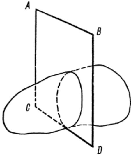
Рис. 1. К определению центра тяжести тела
