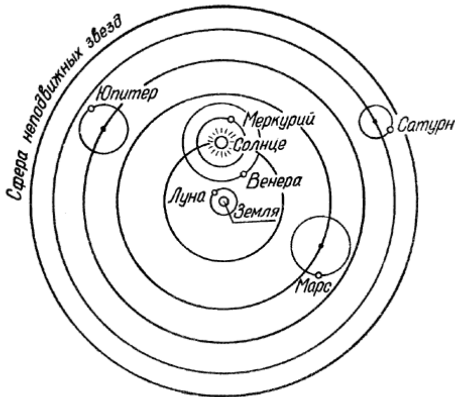
Рис. 4. Эпициклическая система мира
