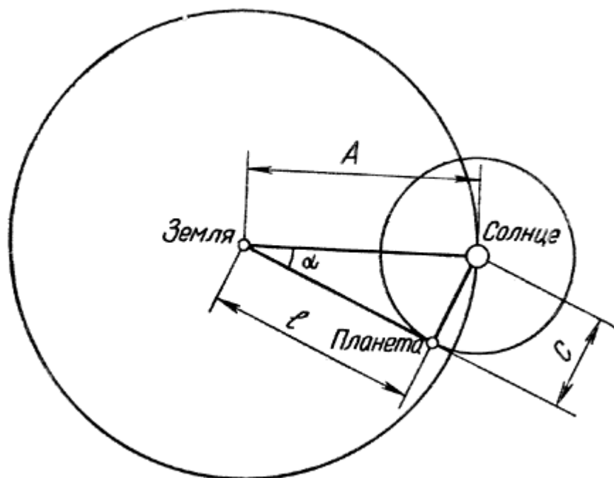
Рис. 5. Схема определения относительного радиуса орбиты планеты
