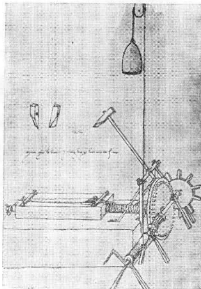
Устройство для насечки напильников.
