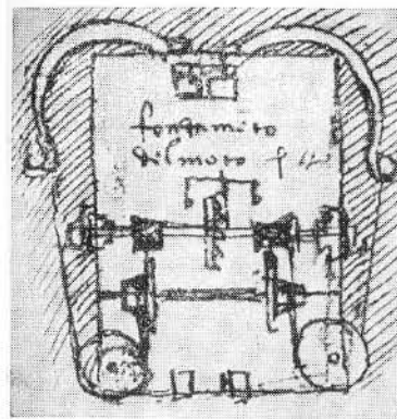
Двигатель, использующий энергию взведенных пружин.
