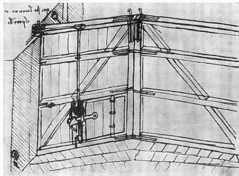
Ворота шлюза.
