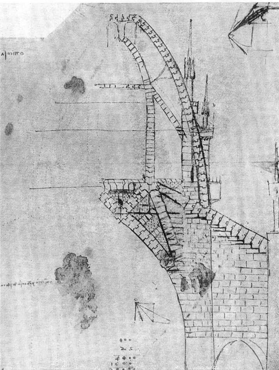
Разрез барабана и купола Миланского собора.
