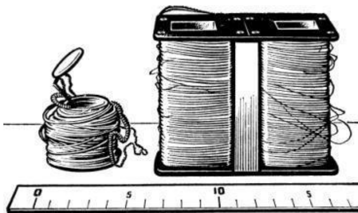
Рис. 11. Катушка и электромагнит собрания приборов, изготовленных Омом.
