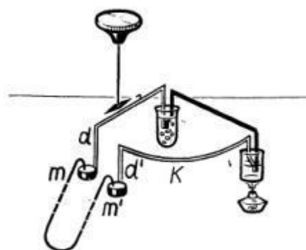
Рис. 4. Электрическая часть установки Г. С. Ома.
