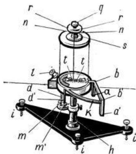
Рис. 3. Схема установки Г. С. Ома.
