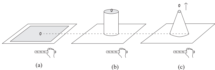
Рис. 9.11: (а) Электризованная линейка под листом бумаги. (б) под бумажным цилиндром. (в) под бумажным конусом. Кусочки бумаги не перемещаются в (а) и (б), но сбрасываются с конуса в положении (с).
