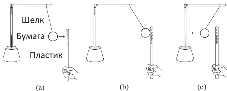
Рис. 4.11: (а) Бумажный диск изначально притягивается потертым пластиком, (б) касается его и затем (с) отталкивается соломой.
