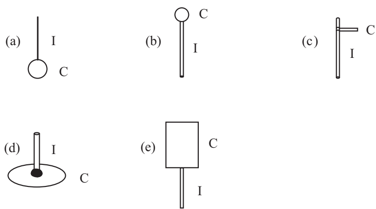
Рис. 2.15: Коллекторы зарядов, состоящие из проводящей части C и изолирующей ручки I.
