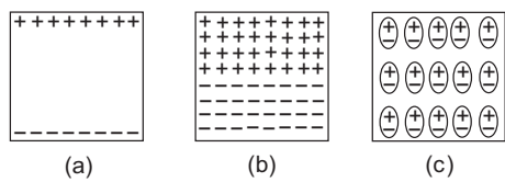
Рис. 13.5: Поляризованные электреты. (a) С реальными и противоположными поверхностными зарядами. (b) С противоположными действительными зарядами, распределенными в объеме диэлектрика. (в) Содержащие ориентированные молекулярные диполи.
