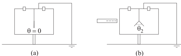
Рис. 10.16: (а) Электроскоп заземлен частью A . Первоначально части A и B имеют нулевой потенциал. (б) Когда натертая акриловая линейка приближается к B , полосы поднимаются.
