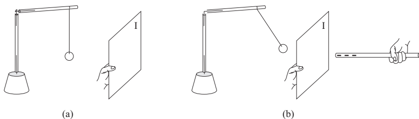
Рис. 8.2: (а) Изолирующий лист из пластика I рядом с разряженным маятником. (б) Диск притягивается натертой соломкой, расположенной с другой стороны пластикового листа.
