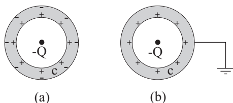
Рис. 8.12: (а) Изолированный проводник c поляризуется из-за наличия внутреннего отрицательного заряда -Q . (б) Заземленный проводник с нейтрализованной внешней стенкой.
