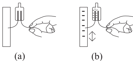
Рис. 11.11: (а) Неоновая лампа не загорается, когда она касается нейтральной акриловой линейки. (б) Потрите одну из его ног отрицательно наэлектризованной линейкой. Обратите внимание, что мигает только электрод, подключенный к линейке.
