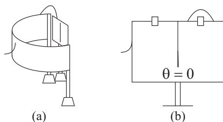
Рис. 10.20: Изолированный электрометр с частями A и B , соединенными проводником (а) Зарядите электрометр, и его внутренняя полоска остается внизу. (б) Электризуйте другую модель электрометра, и его два внутренних листка остаются в нераскрытом состоянии.
