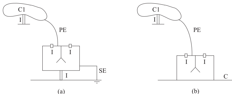
Рис. 10.7: Электрометр с заземленным корпусом. (a) Вторичный электрод подключен к Земле. (b) Корпус на проводящей пластине C , соединенной с землей.
