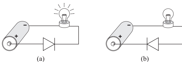
Рис. 3.17: (а) Диод ориентирован вперед и ведет себя как проводник. В этой ориентации возможен поток зарядов. (b) Диод имеет обратную направленность и ведет себя как изолятор. В этой ориентации ток в цепи невозможен.
