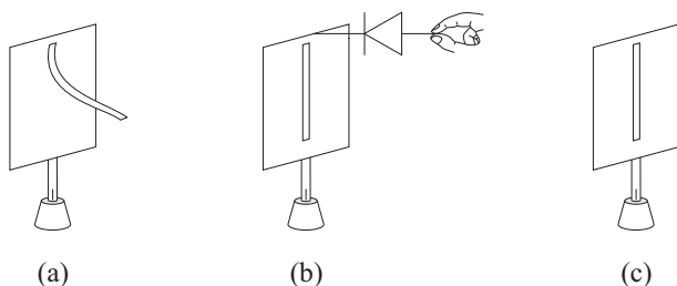
Рис. 3.19: (а) Заряженный электроскоп. (b) Удерживая анод диода в руке, коснитесь катодом картон электроскопа и заметьте, что его полоска сразу падает. (с) Полоска сохраняет вертикальное положение после удаления диода.
