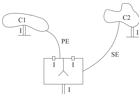
Рис. 10.6: Основной электрод PE соединяет часть A электрометра с проводником C_1 , а вторичный электрод SE соединяет часть B с проводником C_2 .
