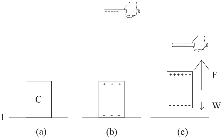
Рис. 4.2: (а) Проводящий кусок бумаги C на изолирующей поверхности I . (b) Макроскопическая поляризация проводника, вызванная присутствием электризованного куска пластика, находящегося рядом с ним. (c) С еще большим приближением пластика, количество поляризованных зарядов на бумаге увеличивается. Если сила F , которую оказывает электризованный пластик на макроскопически поляризованную проводящую бумагу, больше, чем вес W бумаги, она будет притягиваться к пластику.
