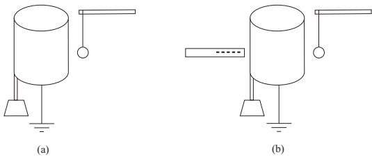
Рис. 8.9: Механизм ПКО не работает, когда натертая акриловая линейка приближается к другой стороне изначально заземленной цилиндрической оболочки.
