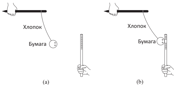
Рис. 4.15: (а) Заземленный диск положительно электризован вблизи отрицательной соломы. (б) Заземленный проводник остается положительно электризованным вблизи соломы, будучи притянутым отрицательными участками изолирующей соломы.
