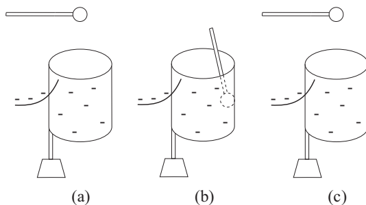
Рис. 7.6: (а) Разряженный коллектор и отрицательно электризованная цилиндрическая оболочка. (б) Прикоснитесь шариком из алюминиевой фольги к внутренней стенке цилиндрической оболочки. (с) Удалив коллектор заряда, убедитесь, что он остается разряженным.
