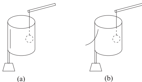
Рис. 7.20: (а) Изолированная цилиндрическая оболочка с внутренним электрическим маятником. (б) Бумажный диск не испытывает влияния при электризации цилиндрической оболочки.
