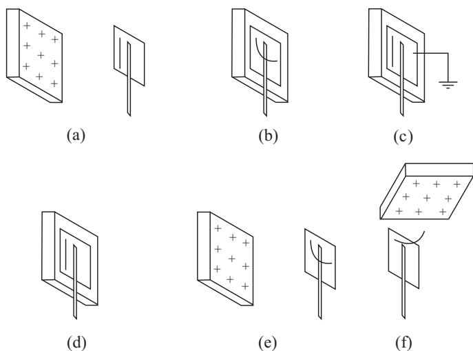
Рис. 6.5: (а) Электризованное основание и сборщик зарядов электрофора, имеющего полоску из папиросной бумаги. (b) Полоска поднимается, когда картон касается электризованной пластины. (с) Полоска падает во время заземления. (d) Она остается в висячем положении, когда заземление отсутствует. (e) Она поднимается, когда сборщик отходит от базы. (f) Полоска, притягиваемая электризованной пластиной.
