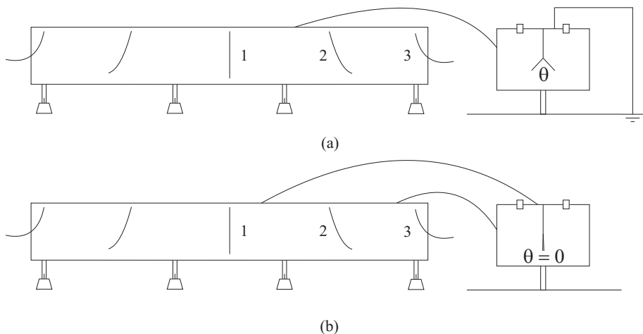
Рис. 10.14: (а) Электроскоп заземлен в точке A и показывает один и тот же угол раскрытия \theta , независимо от места, где подключен вторичный электрод. (б) Изолированный электроскоп с участком A , соединенным с одной точкой наэлектризованного прямоугольника, в то время как участок B соединен с другой точкой прямоугольника. Угол раскрытия электроскопа отсутствует.
