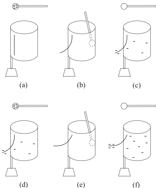
Рис. 7.13: (а) Цилиндр с разряженным и электризованным коллектором. (b) Коснитесь заряженным коллектором внутреннюю стенку цилиндра. Эту процедуру можно повторить много раз. (с) - (f): коллектор полностью разряжается после каждого контакта, в то время как цилиндр становится все более и более электризованным.
