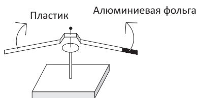
Рис. 2.8: Версориум Дюфе.
