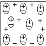
Рис. 13.6: Общий электрет.
