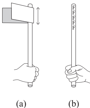
Рис. 1.2: (а) Пластиковая солома, потертая бумагой. (б) Буква F представляет потертую область соломы.
