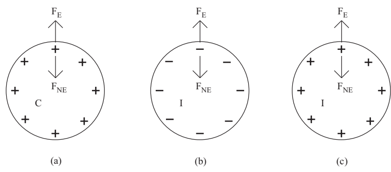
Рис. 14.2: (а) Проводящая сфера C положительно электризована. (b) Изолирующая сфера I отрицательно электризована. (в) Изолирующая сфера I положительно электризована.
