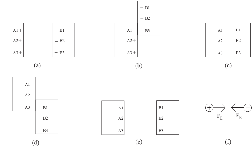
Рис. 14.11: (a) Гипотетическая нейтрализация двух противоположно электризованных изоляторов A и B . (b) Нейтрализация точек A1 и B3 во время их контакта. (c) Нейтрализация точек A2 и B2 во время их контакта. (d) Нейтрализация точек A3 и B1 во время их контакта. (e) Изоляторы остаются нейтральными после разделения. (f) Электростатические силы притяжения, F_E , действующие между противоположно электризованными частицами.
