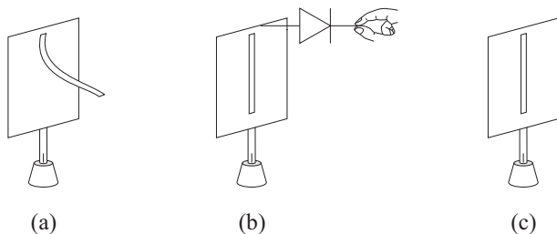
Рис. 3.18: (а) Заряженный электроскоп. (b) Удерживая катод диода в руке, коснитесь анодом картон электроскопа и обратите внимание, что его полоска сразу падает. (с) Полоска остается в висячем положении после удаления диода.
