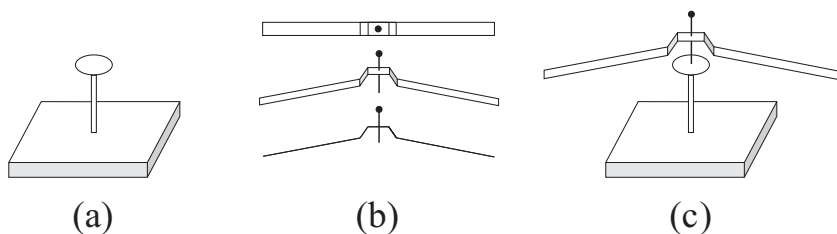
Рис. 2.7: Пластиковый версориум со штифтом, установленным в центре непроводящей полосы. (а) Фиксированное основание версориума. (б) Шляпа версориума (пластиковая полоса) с прикрепленным к ней штифтом. с) Версориум в собранном виде.
