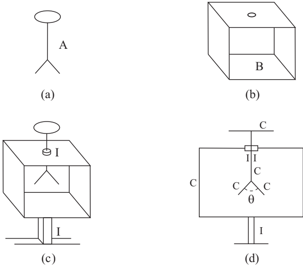
Рис. 10.1: Электроскоп с токопроводящим корпусом. (а) Проводящая часть A . (b) Проводящая часть B . (в) Вид спереди. Между частями A и B имеется изолятор I . Есть еще один изолятор I между частью B и землей. (d) Вид инструмента сбоку. Буквами C обозначены проводники, буквами I — изоляторы, а буквой \theta обозначен угол раскрытия между подвижными листьями.
