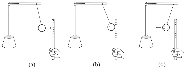
Рис. 4.12: (a) Проводящий диск поляризуется находящейся рядом электризованной соломой. Между ними возникает притяжение. (b) Во время контакта происходит обмен электризованных частиц. В результате этого обмена диск становится электризованным с суммарным зарядом того же знака, что и соломка. (c) Электризованный диск затем отталкивается соломой.
