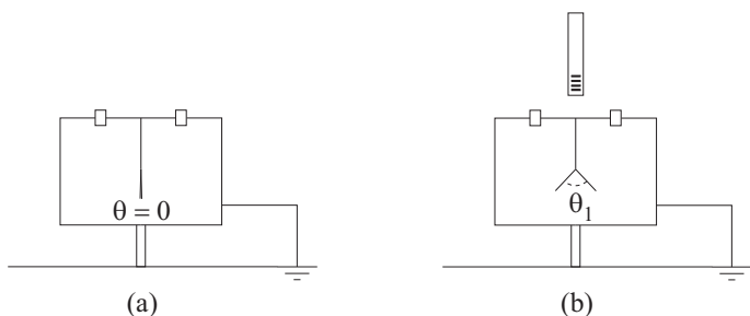
Рис. 10.15: Электроскоп заземлен частью B . (а) Части A и B изначально имеют нулевой потенциал. (б) Когда натертая акриловая линейка приближается к части A , полосы поднимаются.
