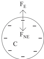
Рис. 14.1: Сферический проводник C равномерно электризован. Мы показываем суммарную отталкивающую электростатическую силу F_E , действующую на верхний отрицательный заряд со стороны всех других отрицательных зарядов, и силу неэлектростатического происхождения, F_{NE} , ответственную за удержание этого верхнего заряда в покое на поверхности сферы.
