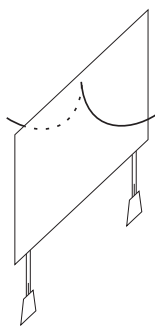
Рис. 7.3: Электризованный прямоугольник.
